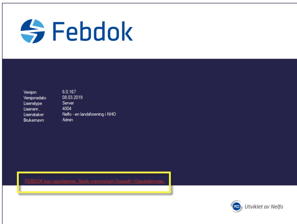
Figur 1 Oppstartsskjerm
